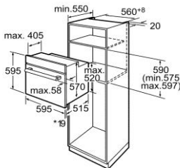
*Bei Metallfronten 20mm Maße in mm
