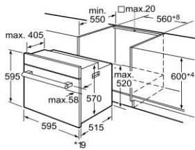
*Bei Metallfronten 20mm Maße in mm
