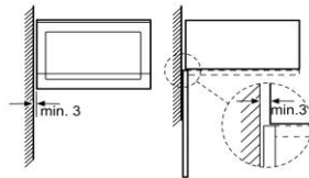
Maße in mm
