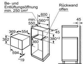
Be- und Entlüftungöffnung min. 250 cm 2 * 20 mm für Metallfront Maße in mm
