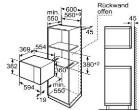
* 20 mm für Metallfront Maße in mm
